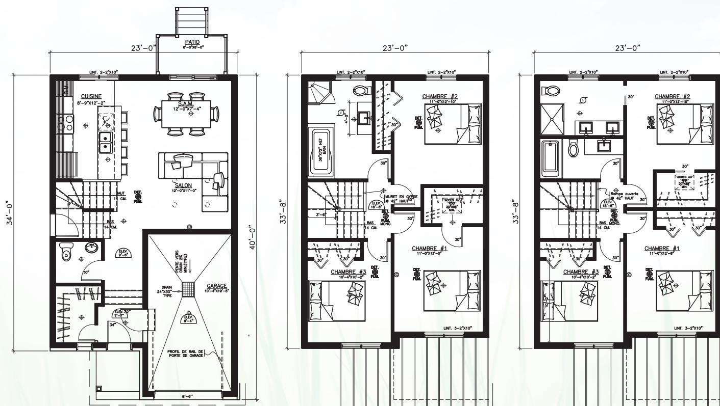
REZ-DE-CHAUSSÉE 23'
