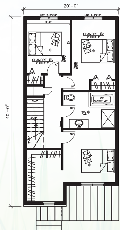
ÉTAGE 20' (1-SDB)
