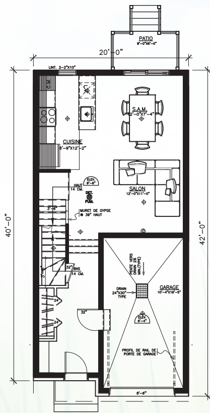
REZ-DE-CHAUSSÉE 20' de BASE
