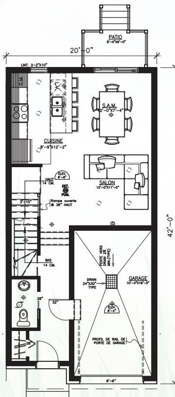
REZ-DE-CHAUSSÉE 20'
